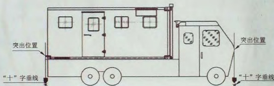
图 A.1 车辆前后突出位置标注示意
